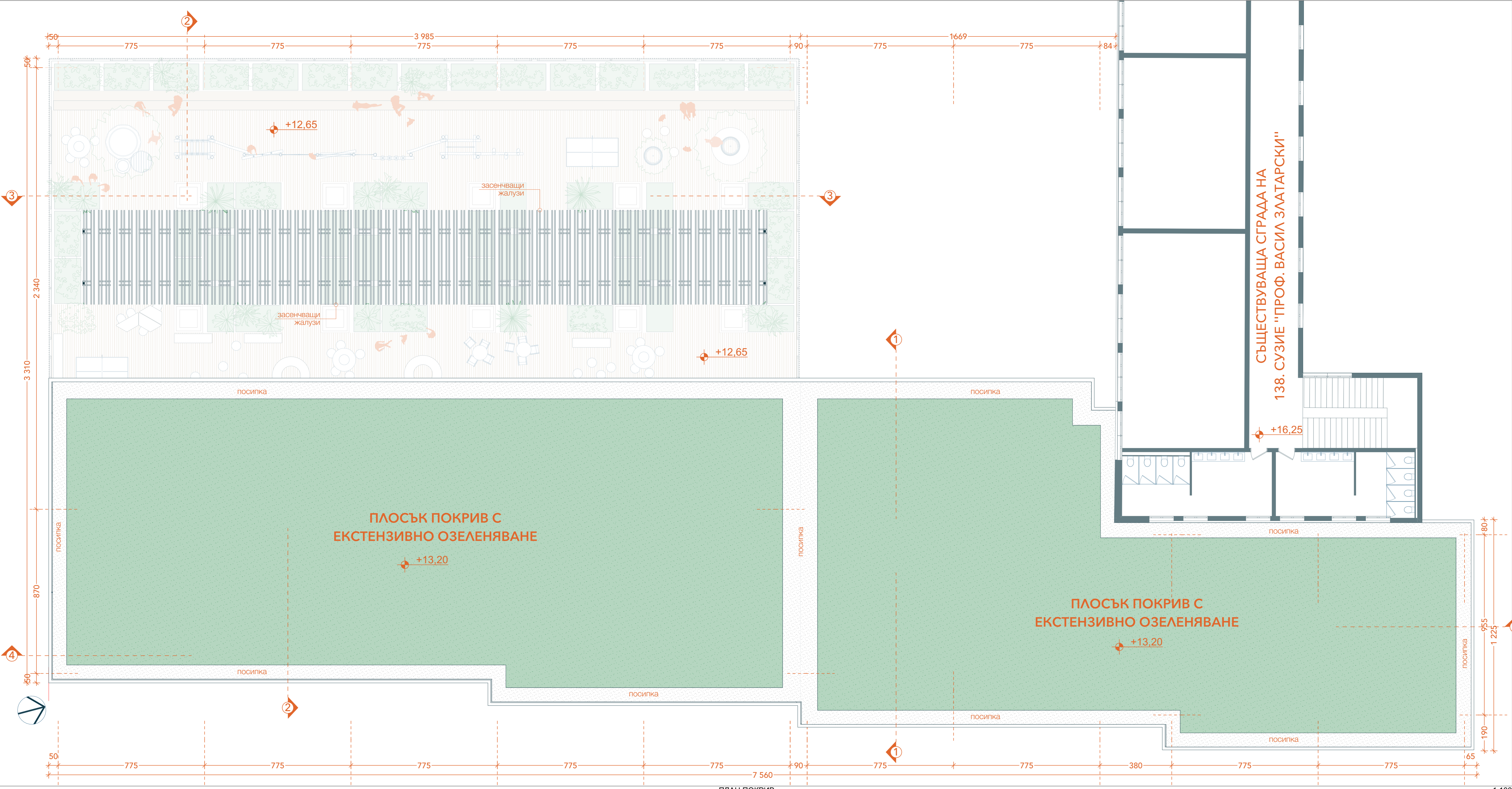
ПЛАН ПОКРИВ
