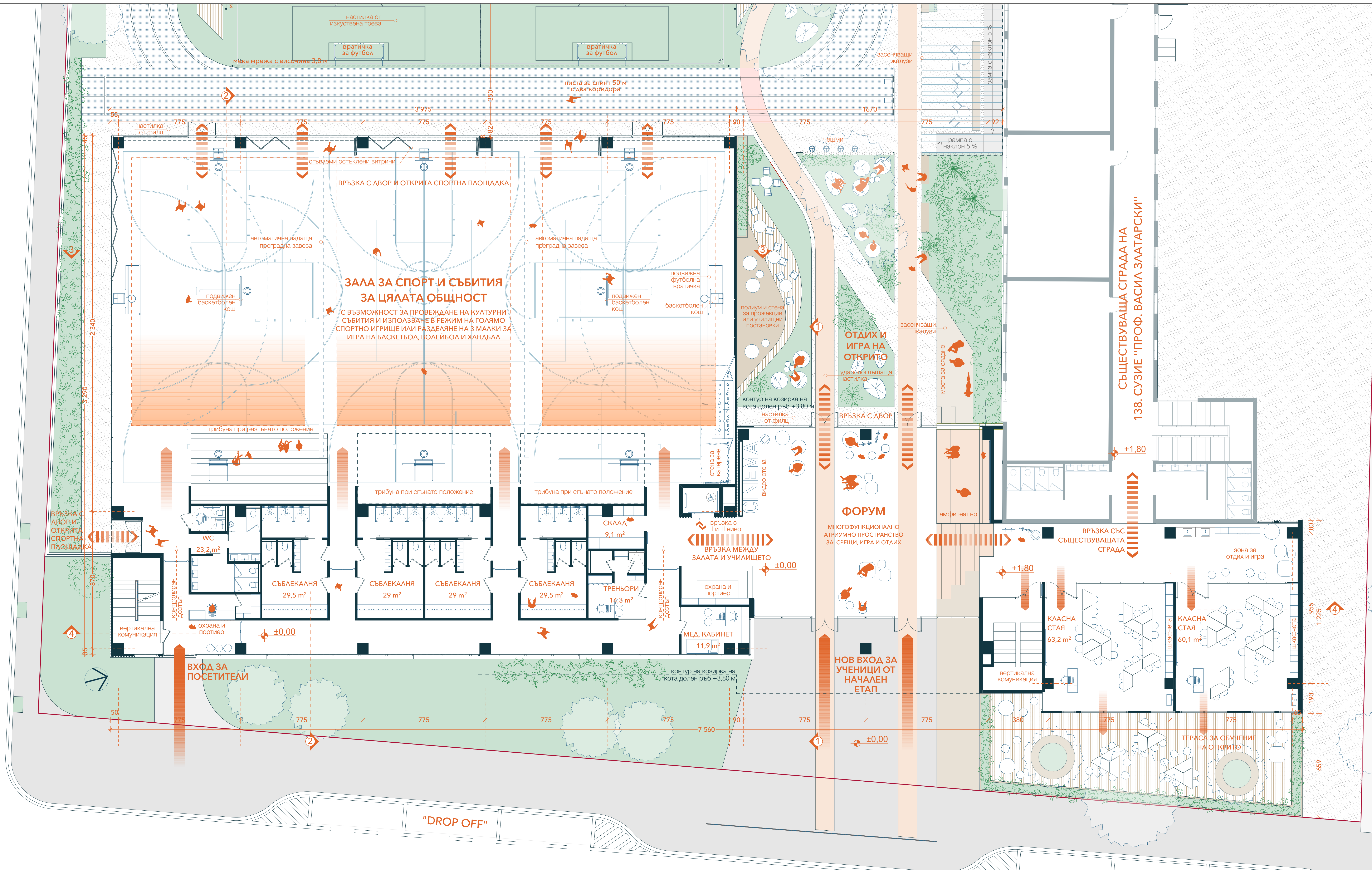
РАЗПРЕДЕЛЕНИЕ КОТА ±0.00
